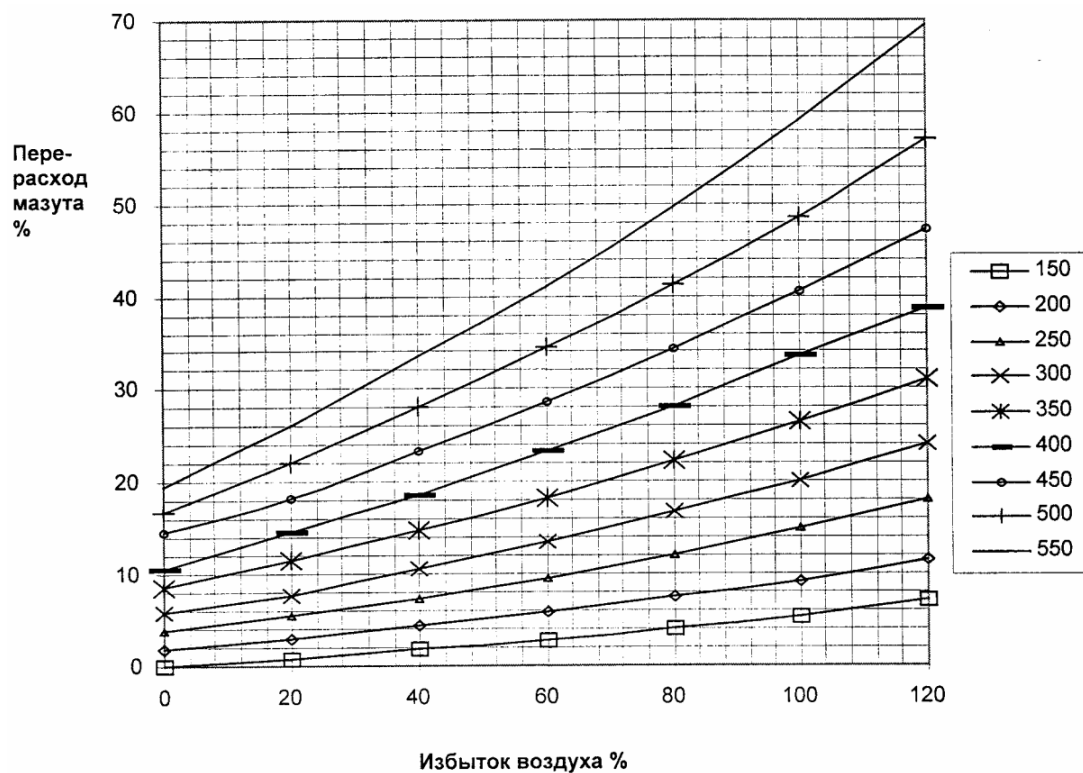
Рис. 14 Влияние избытка воздуха на перерасход мазута (справа - температура уходящих газов °C). Базовое топливо – C_4H_5 , t_{ух.газов} - 150°C, избыточный воздух = 94,5 \cdot O_2 / (21 - O_2) , базовый КПД - 89,93%
