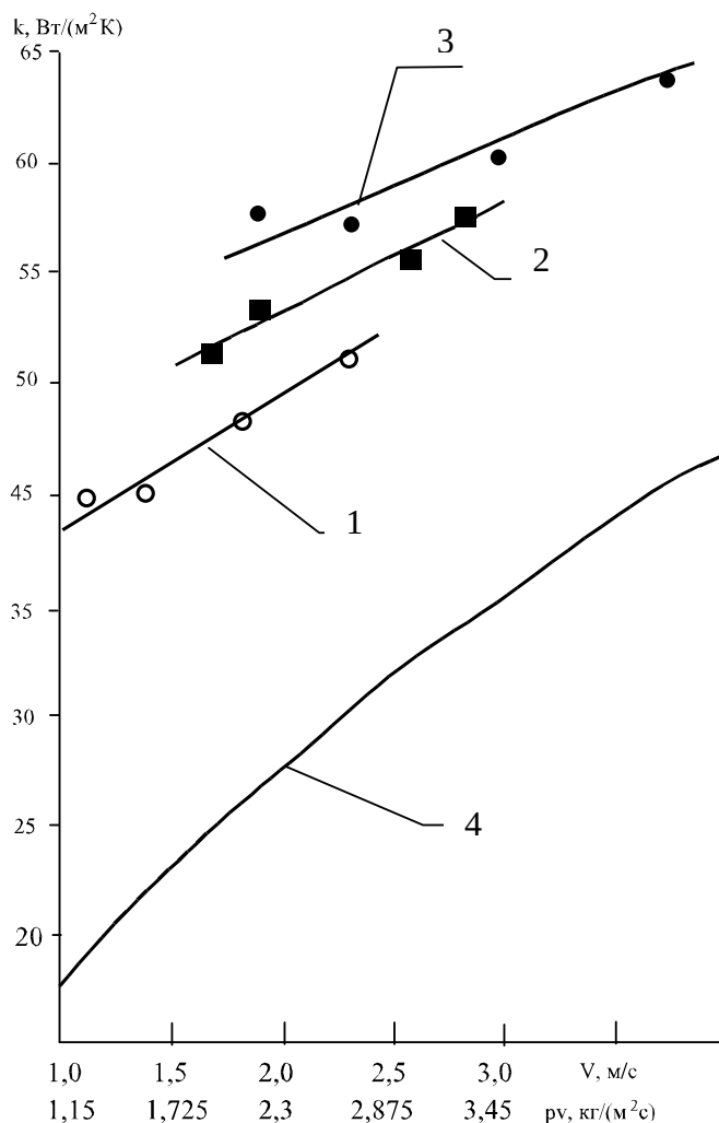
Рис. 7. Зависимость коэффициента теплопередачи k от скорости газов v и плотности орошения V 1 – V = 2,28 \div 3,57 кг/м²·с; 2 – V = 2,83 \div 3,67 кг/м²·с; 3 – V = 3,19 \div 4,03 кг/м²·с; 4 – для воздуха («сухой» теплообмен)
