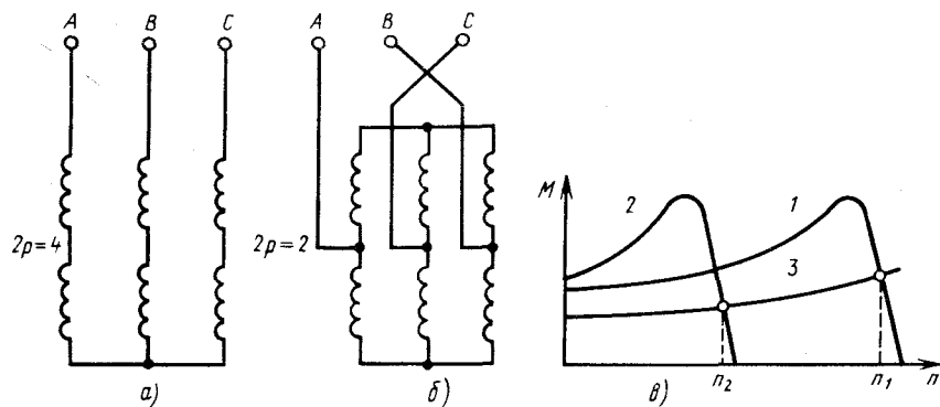
Рис. 57. Двухскоростной электродвигатель:
