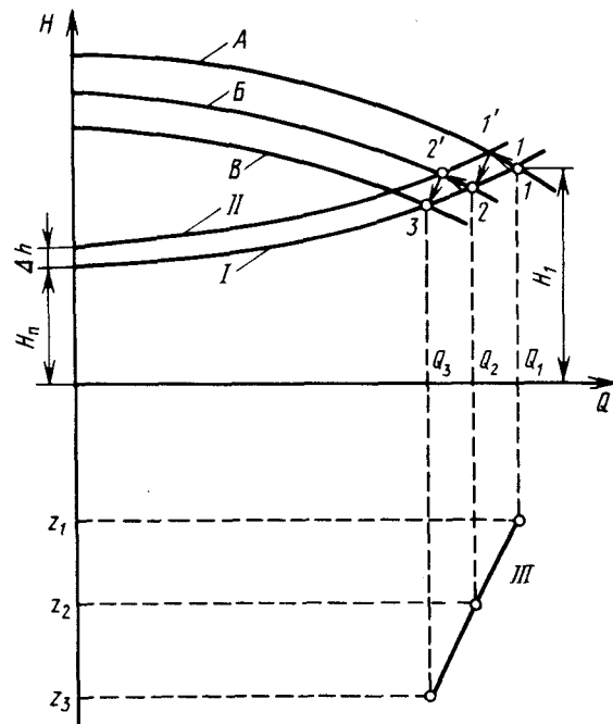
Рис. 75. Процесс стабилизации уровня жидкости в резервуаре:
