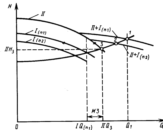
Рис. 71. Образование мертвых зон (МЗ) в процессе регулирования насосной установки:
