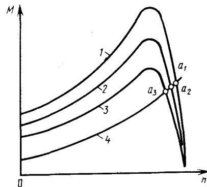
Рис. 55. Механические характеристики электродвигателя при изменении напряжения:
