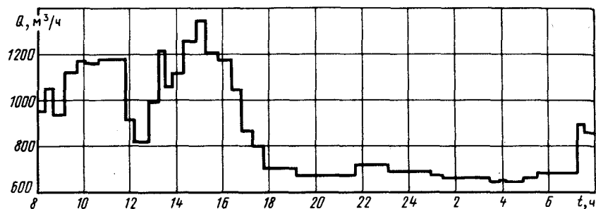
Рис. 14. Суточный график водоподачи насосной установки свиноводческого промышленного комплекса
