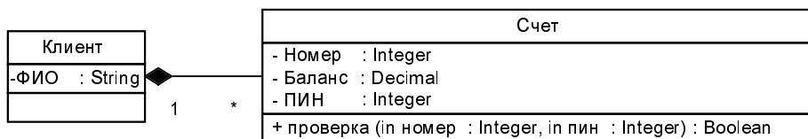
Рис. Д.6. Пример диаграммы классов унифицированного языка моделирования UML
