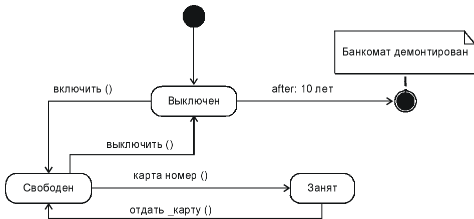
Рис. Д. 11. Пример диаграммы состояний унифицированного языка моделирования UML
