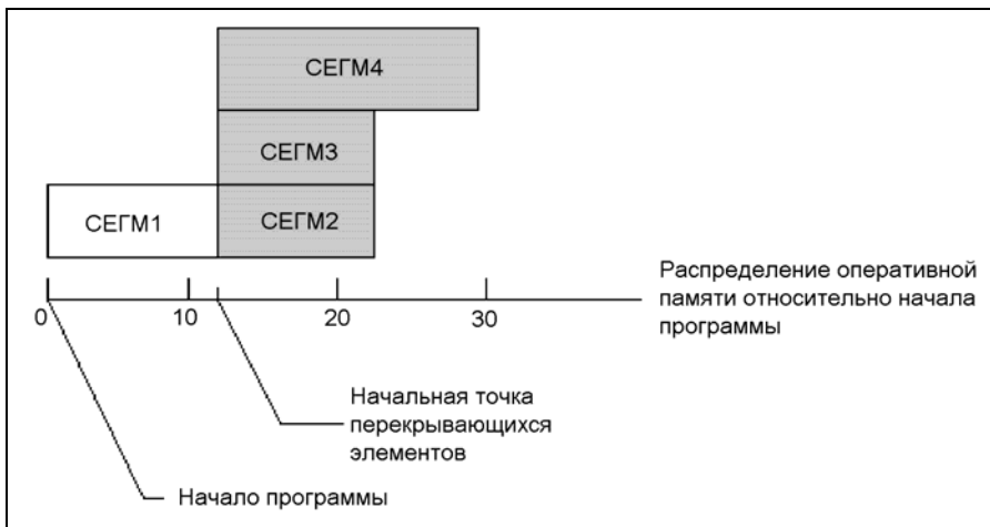
Рис. О.2. Схема распределения памяти с использованием оверлейной структуры
