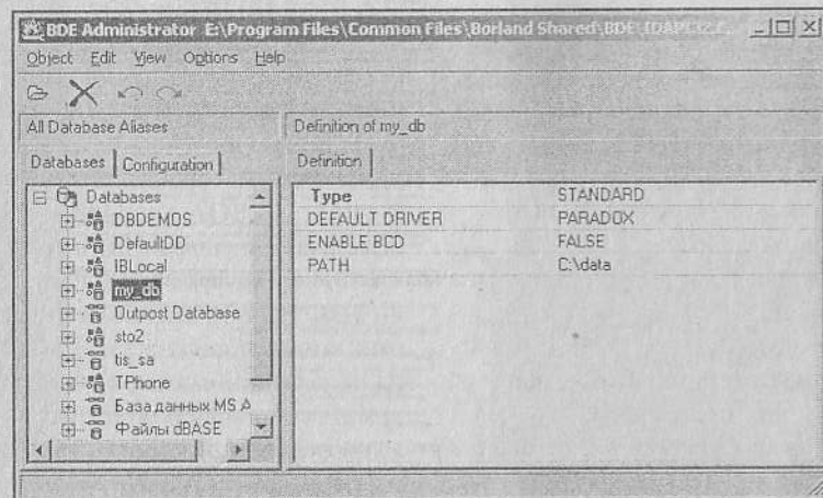
Рис. А.10. Программа BDE Administrator — просмотр псевдонимов
