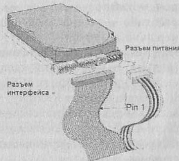
Рис. А.16. Интерфейс ATA — подключение жесткого диска
