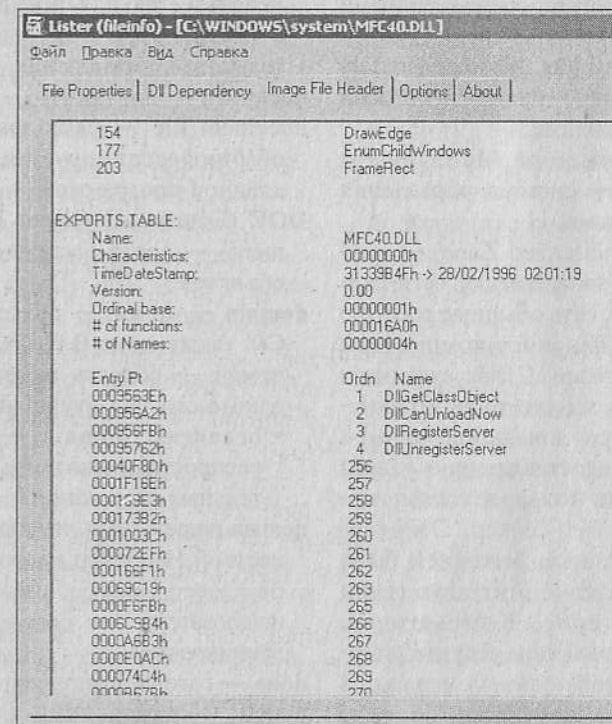
Рис. D.1. Информация о DLL
