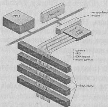
Рис. Е.4. Внутреннее устройство шины EISA
