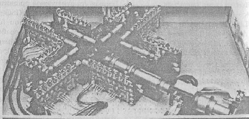
Рис. О.1. Оптический компьютер DOC-II
