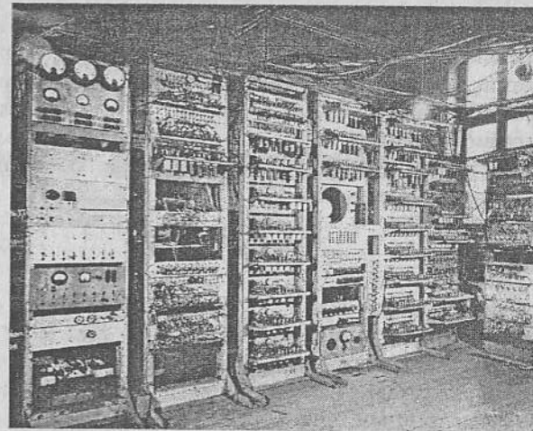
Рис. В.5. Компьютер Mark II
